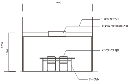
■立面図
